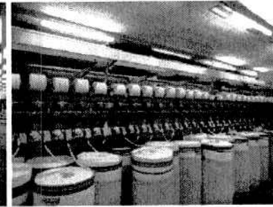
FILATÓRIO N.1
